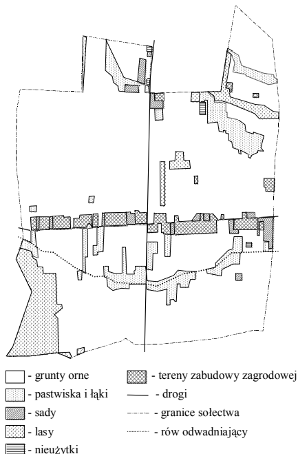
Ryc. 1. Struktura użytkowania ziemi w sołectwie Kromolin Stary.
